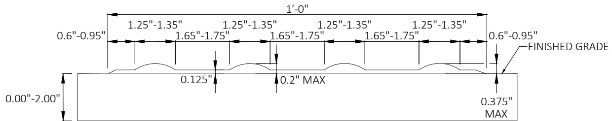
SECTION A-A
